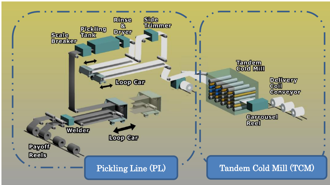
fig. 1. PLTCM Layout
